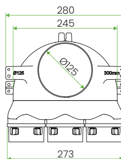
wersja podłogowa
