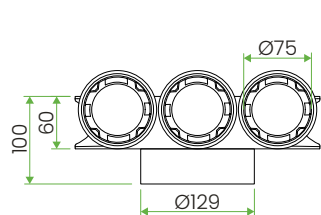
wersja sufitowa
