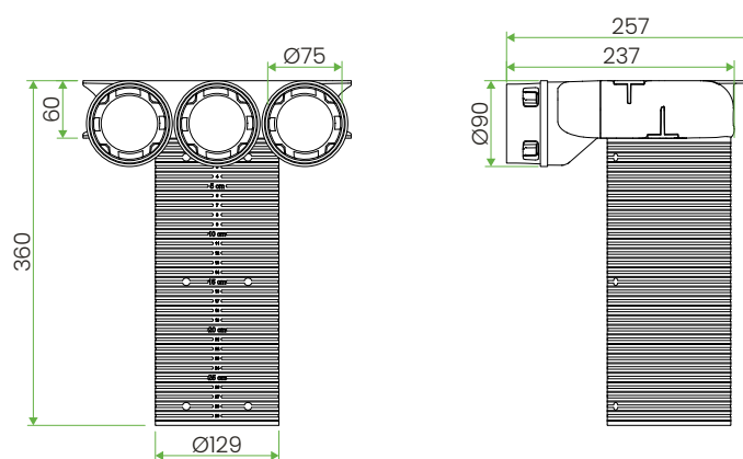
wersja sufitowa
