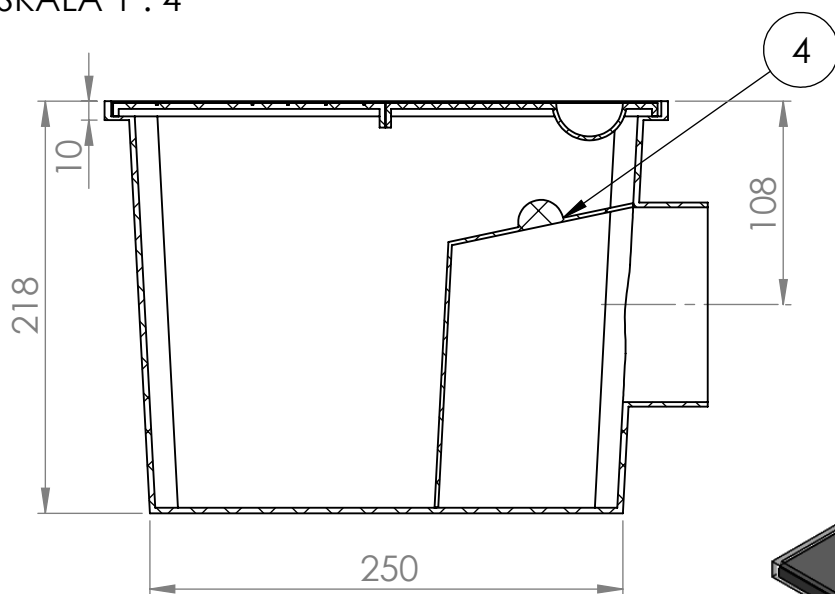
PRZEKRÓJ A-A SKALA 1 : 4
