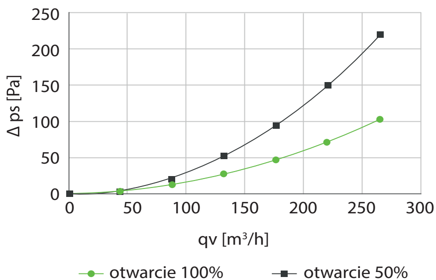
Nawiewna charakterystyka aerodynamiczna anemostatów PEFLEX PREMIUM Ø125 mm
