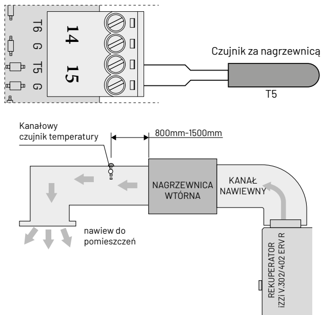
Rys. Schemat podłączenia czujnika temperatury za wodną nagrzewnicą wtórną.
