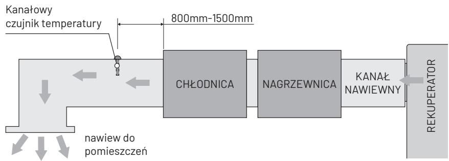
Rys. Schemat umiejscowienia czujnika przy jednoczesnym podłączeniu chłodnicy i nagrzewnicy wtórnej
