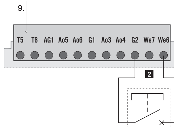
Rys. Schemat podłączenia przełącznika funkcji kominek (dzwonek - impulsowy)
