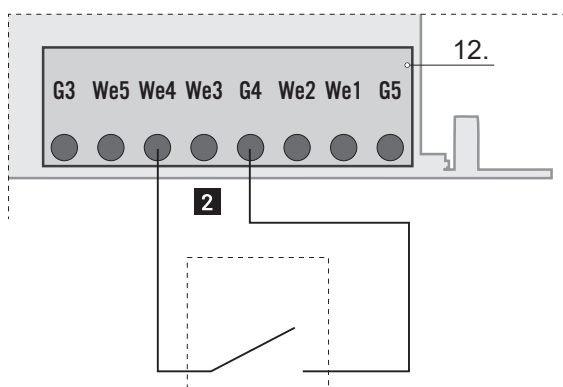
Rys. Schemat podłączenia styku z centrali PPOŻ (zatrzymanie pracy centrali)
