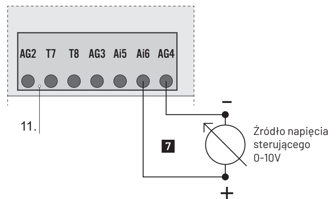
Rys. Schemat podłączenia sygnału 0-10V
