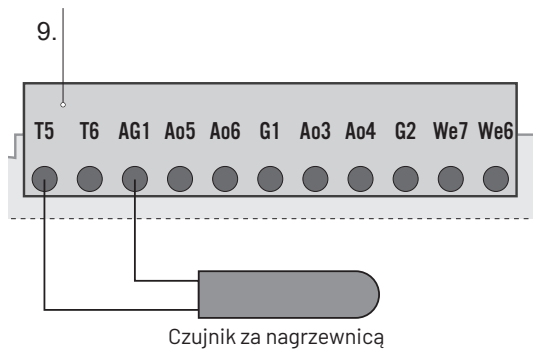
Rys. Schemat podłączenia czujnika
