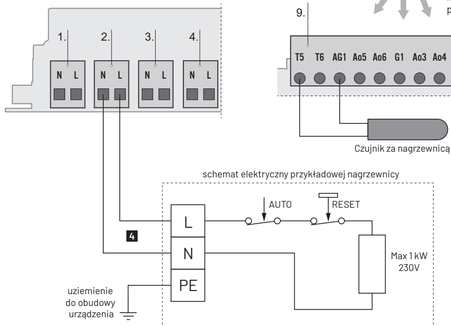
Rys. Schemat podłączenia wtórnej nagrzewnicy elektrycznej 1-fazowej on/off o mocy do 1,0 kW.
